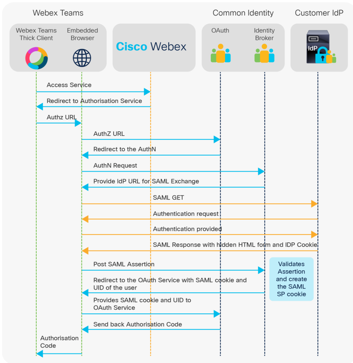
図 1. Cisco Webex プラットフォームを使用した認証と認可のフロー
