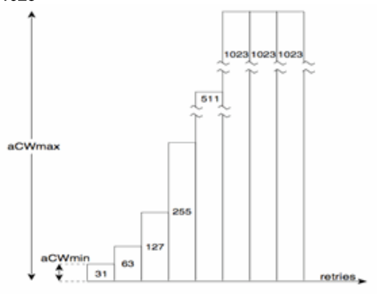
Figure 7 - Pour 802.11b/g CWmin = 31, pour 802.11a CWmin = 15, tous deux ont un CWmax de 1023
