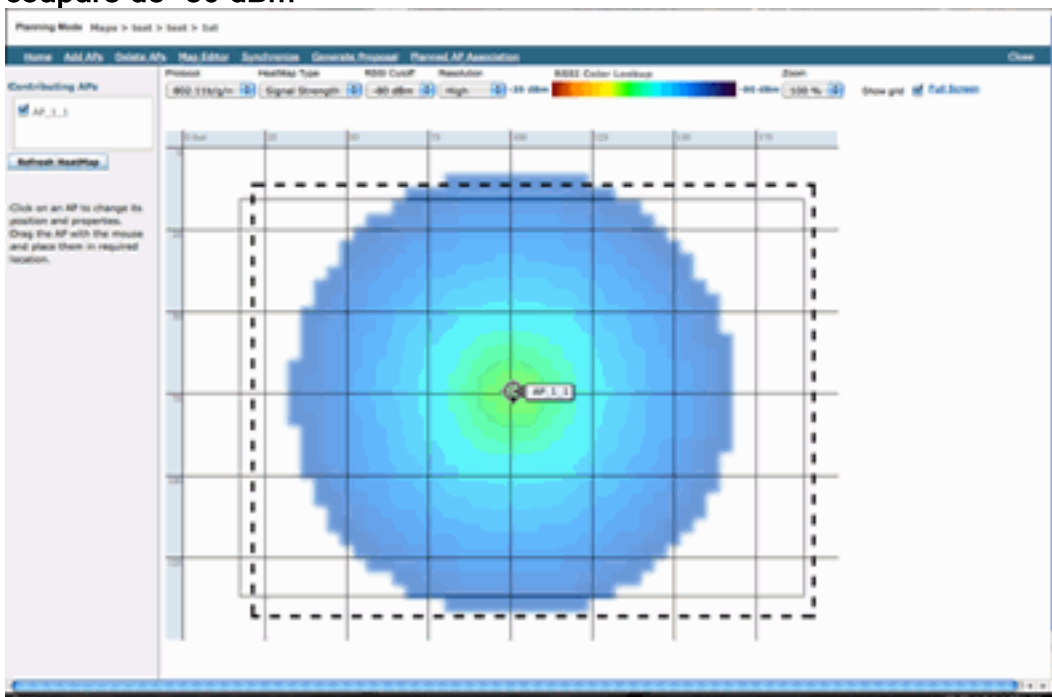
Figure 12 : Exemple de couverture de CleanAir MMAP avec une alimentation de 1 dBm et une coupure de -80 dBm
