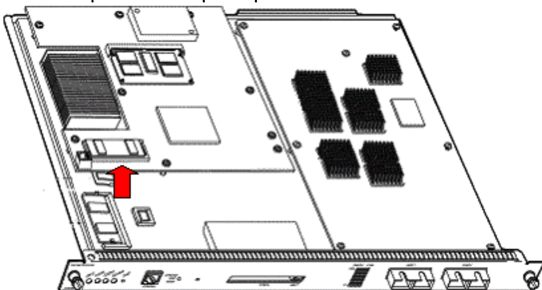
Emplacement du bootflash pour MSFC2 expédié après novembre 2001
