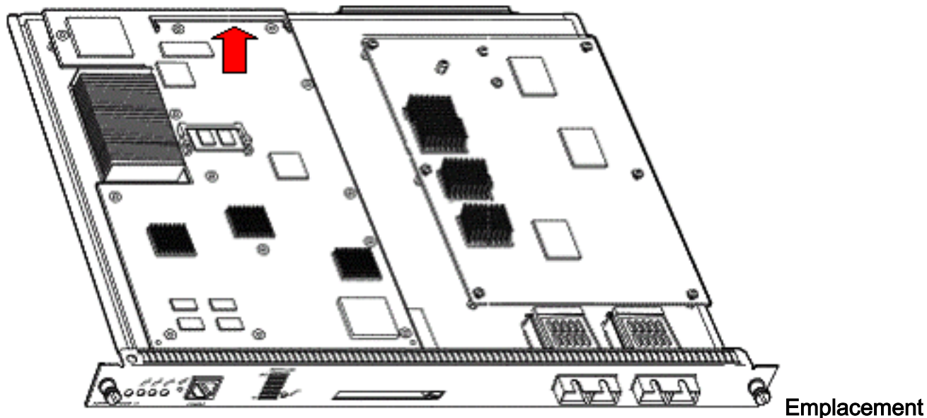
Emplacement du bootflash pour MSFC2 expédié avant novembre 2001
