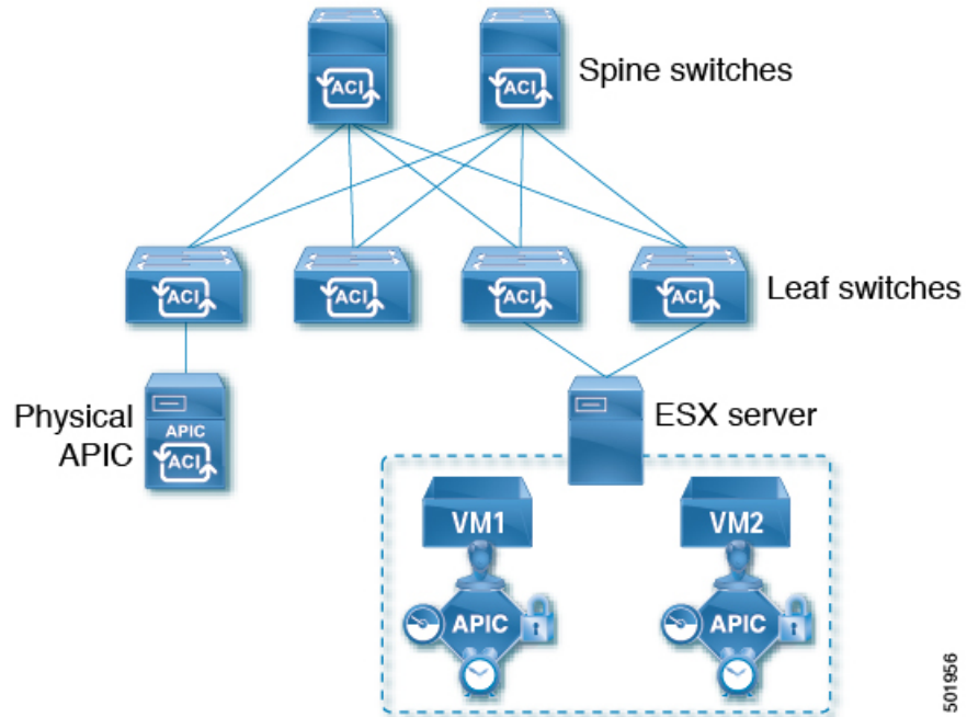
Figure 13: Cisco Mini ACI Fabric
