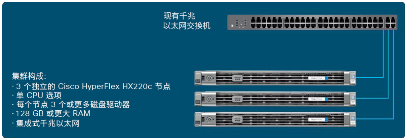
图 1. Cisco HyperFlex Edge
