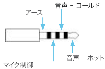
3.5 mm ミニ ジャック、4 極 (マイク)
