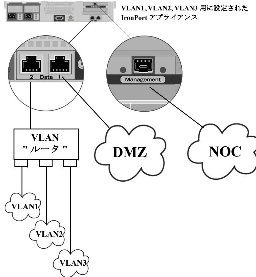
図 36-1 VLAN を使用したアプライアンス上の使用可能なネットワーク数の増加
