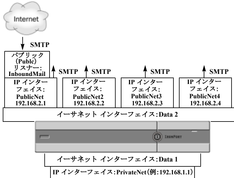
図 23-13 1つのイーサネット インターフェイス上にある4つの Virtual Gateway アドレス
