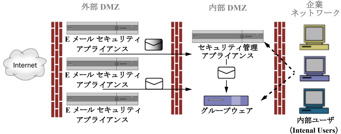
図 41-1 Cisco コンテンツ セキュリティ管理仮想アプライアンスによる一般的なネットワーク設定
