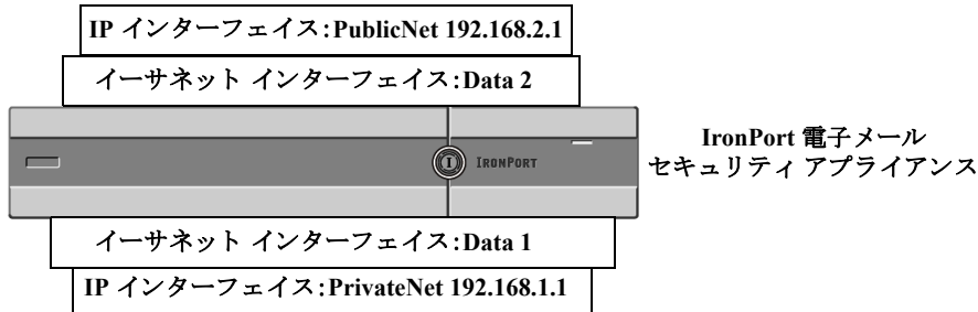
図 23-9 パブリック インターフェイスとプライベート インターフェイスの例
