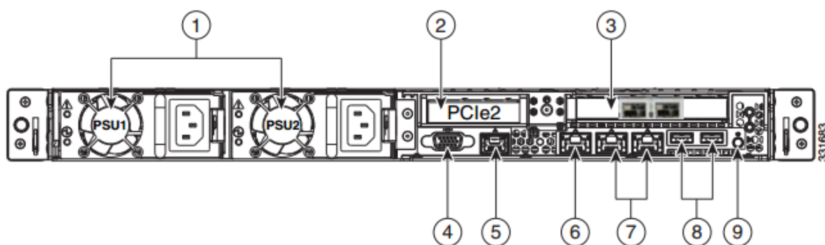
図 4 : Cisco UCS C220 M3 背面の詳細図
