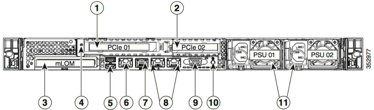
図 6 : Cisco UCS C220 M4 背面の詳細図
