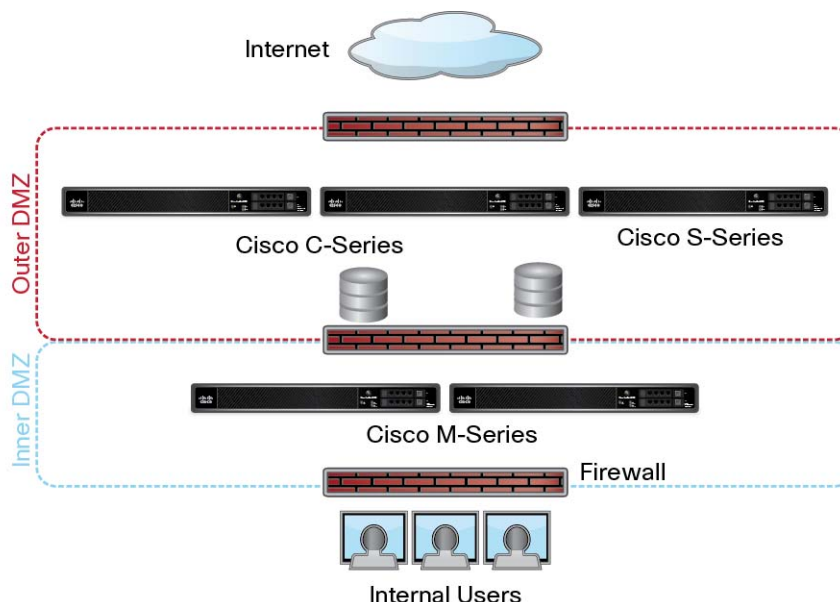
図 2-1 Security Management Applianceを含む一般的なネットワーク設定
