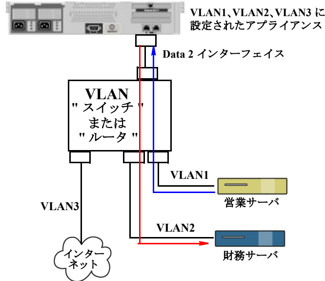
図 37-1 VLAN によるアプライアンス間通信の実現
