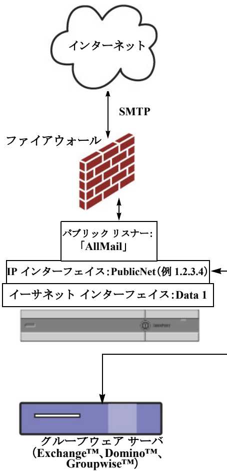
図 3-2 リスナー 1 個の設定
