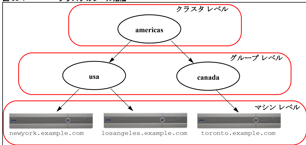
図 39-1 クラスタのレベル階層
