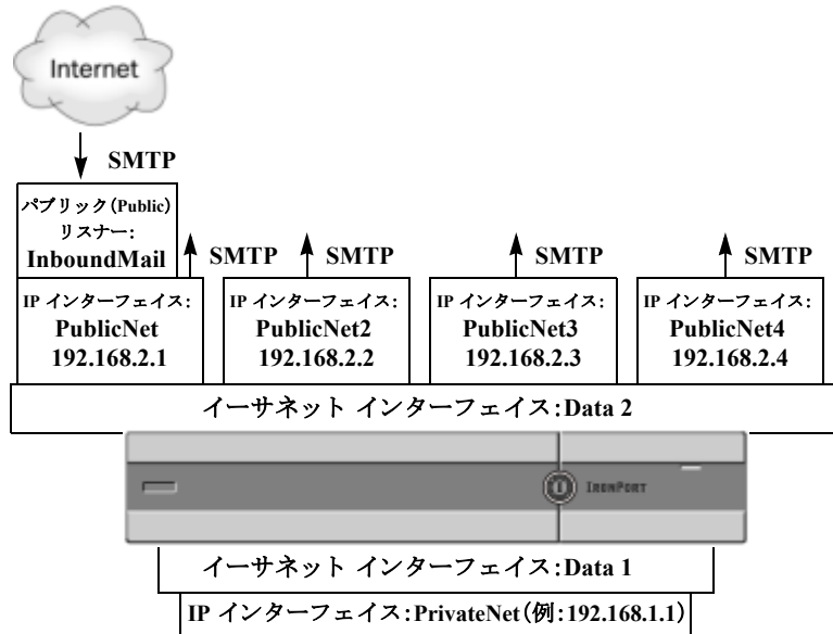
図 25-13 1つのイーサネット インターフェイス上にある4つの Virtual Gateway アドレス
