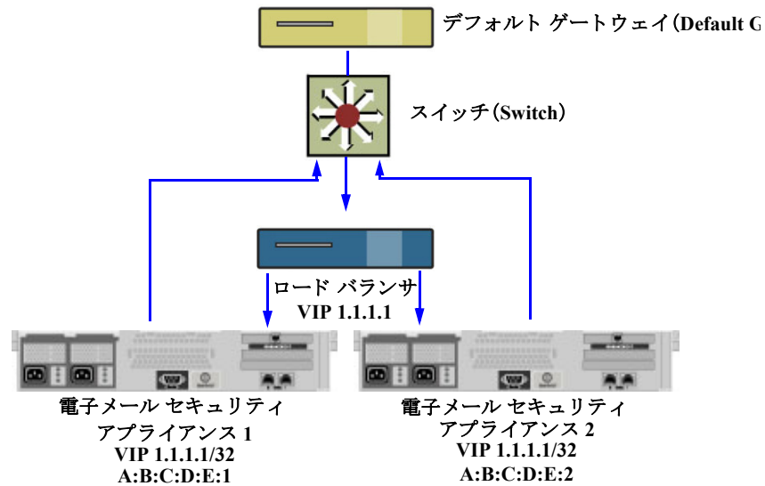
図 37-2 DSR を使用したスイッチ上の複数の E メール セキュリティ アプライアンス間でのロード バランス
