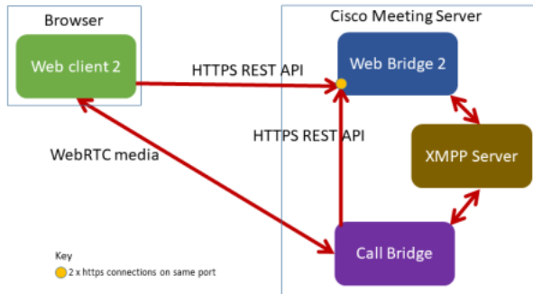
図 1 : Web Bridge 2 のセットアップのフロー図
