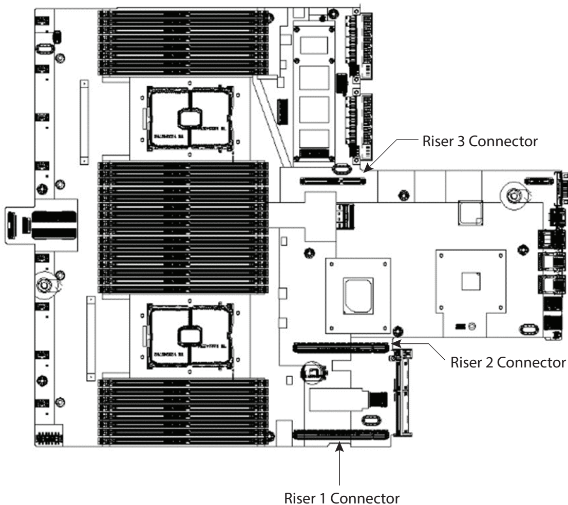
図 16 63HX220C M6 All NVMe/All Flash/Hybrid サーバ ノード ライザー コネクタの場所 HX220 M6 Motherboard
