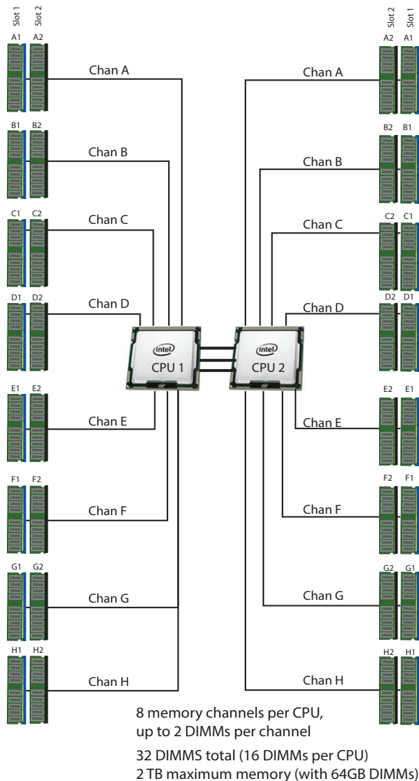
図 8 HX240C M6 All NVMe / All Flash / Hybrid サーバ ノード メモリの構成
