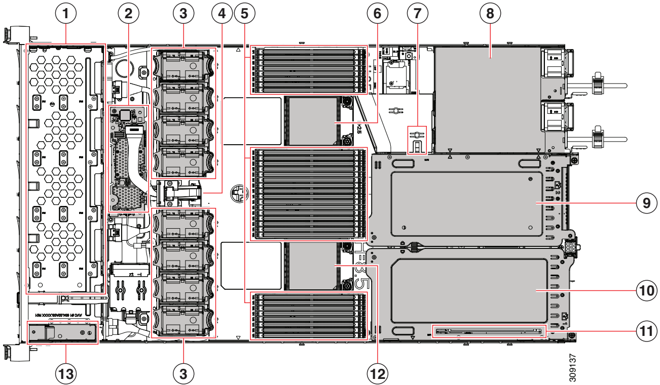
図 14 上部カバーがオフの HX220 M6 All NVMe/All Flash/Hybrid サーバ ノード (フルハイト、フル幅の PCIe カード)
