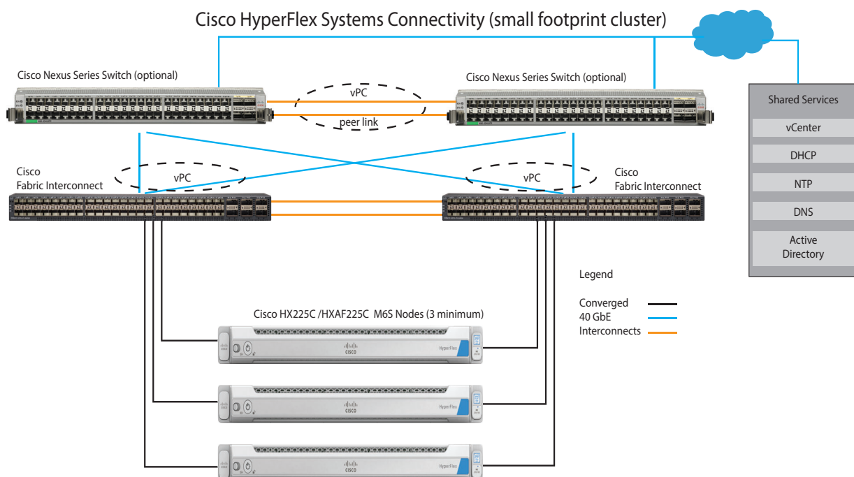
図 9 データセンター ファブリック インターコネクト展開モードの HX220C M6 All NVMe/All Flash/Hybrid サーバー ノードを使用するスモール フットプリント クラスタ。
