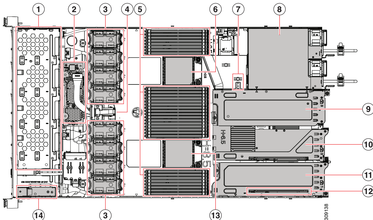
図 15 上部カバーがオフの HX220 M6 All NVMe/All Flash/Hybrid サーバ ノード (フルハイト、ハーフ幅の PCIe カード)
