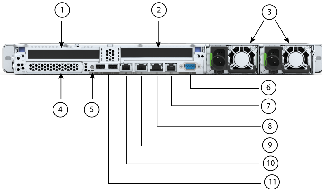
図 7 シャーシ背面図 (フルハイト、長さ 3/4 の PCIe ライザー X 2)
