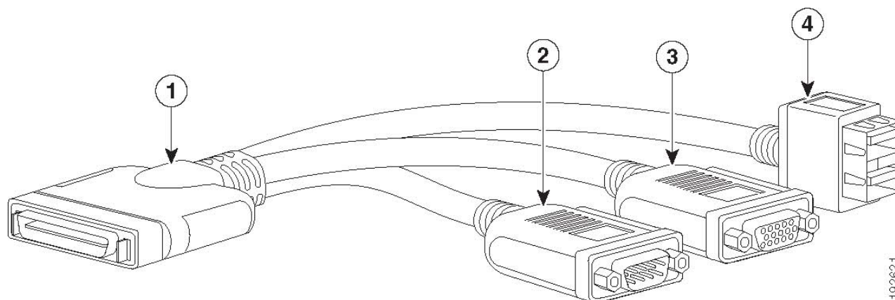
図 20 KVM ケーブル
