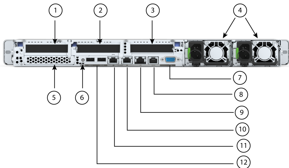
図 6 シャーシ背面図 (3つのハーフハイ ト、長さ 3/4 の PCIe ライザー)
