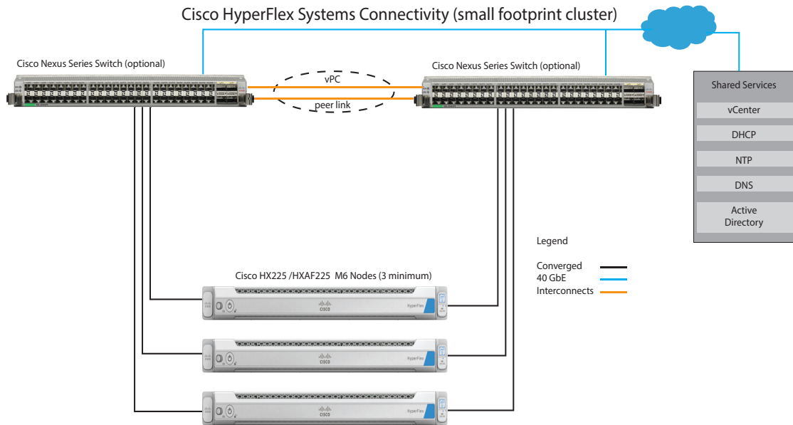
図 10 データセンター ファブリック インターコネクト展開モードの HX220C M6 All Flash/Hybrid サーバー ノードを使用するスモール フットプリント クラスタ。
