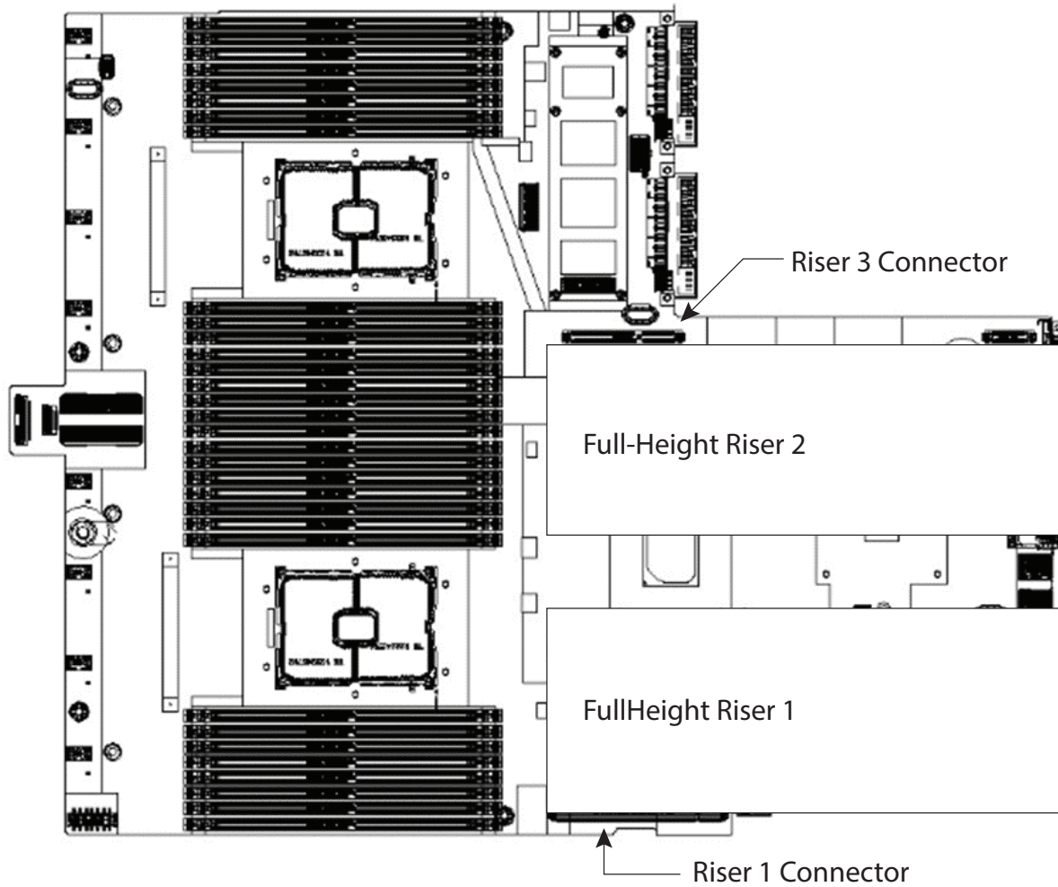
図 18 2つのフルハイト ライザーが接続された HX220 M6 All NVMe/All Flash/Hybrid HX220 M6 Motherboard
