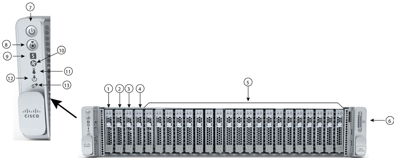
図 4 シャーシ前面図 : HX-E-245-M6SX (Hybrid)
