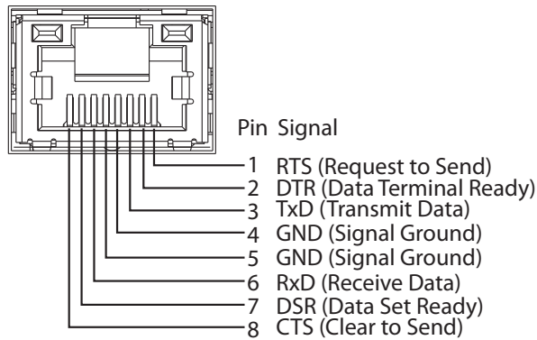
図 25 シリアルポート (RJ-45 のメスコネクタ) のピン割り当て Serial Port (RJ-45 Female Connector)
