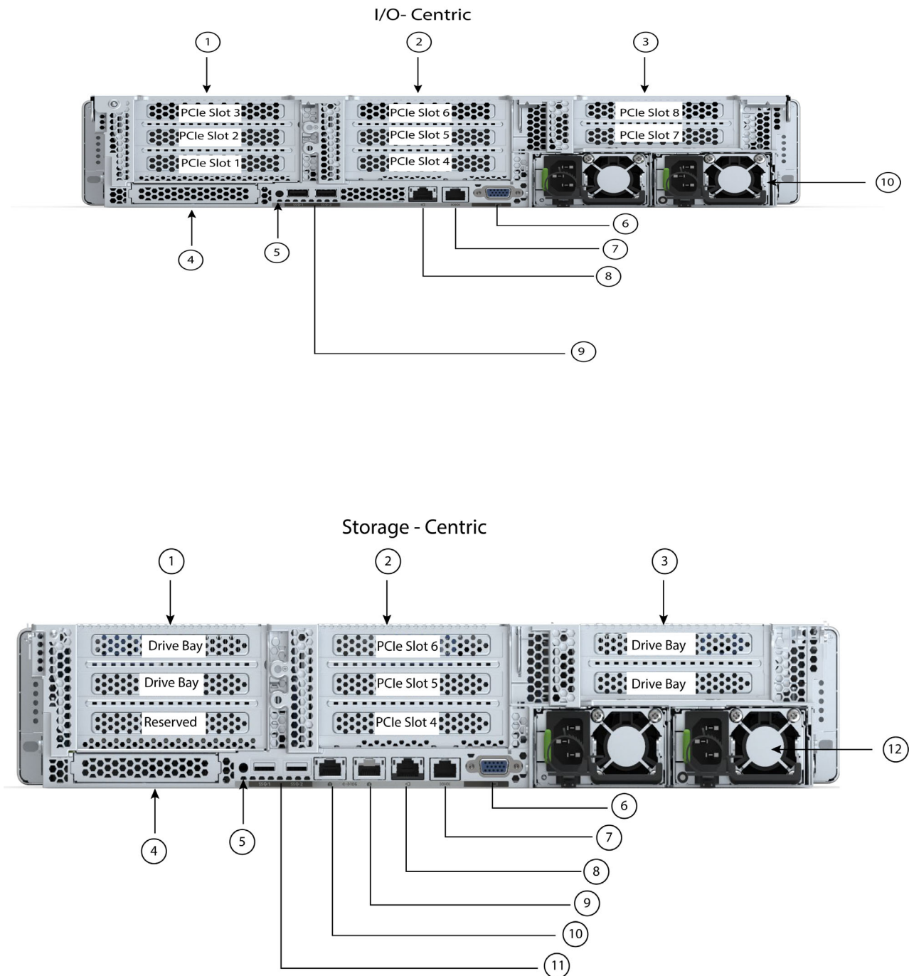
図 5 シャーシ背面図 : HX-E-245-M6SX (Hybrid)
