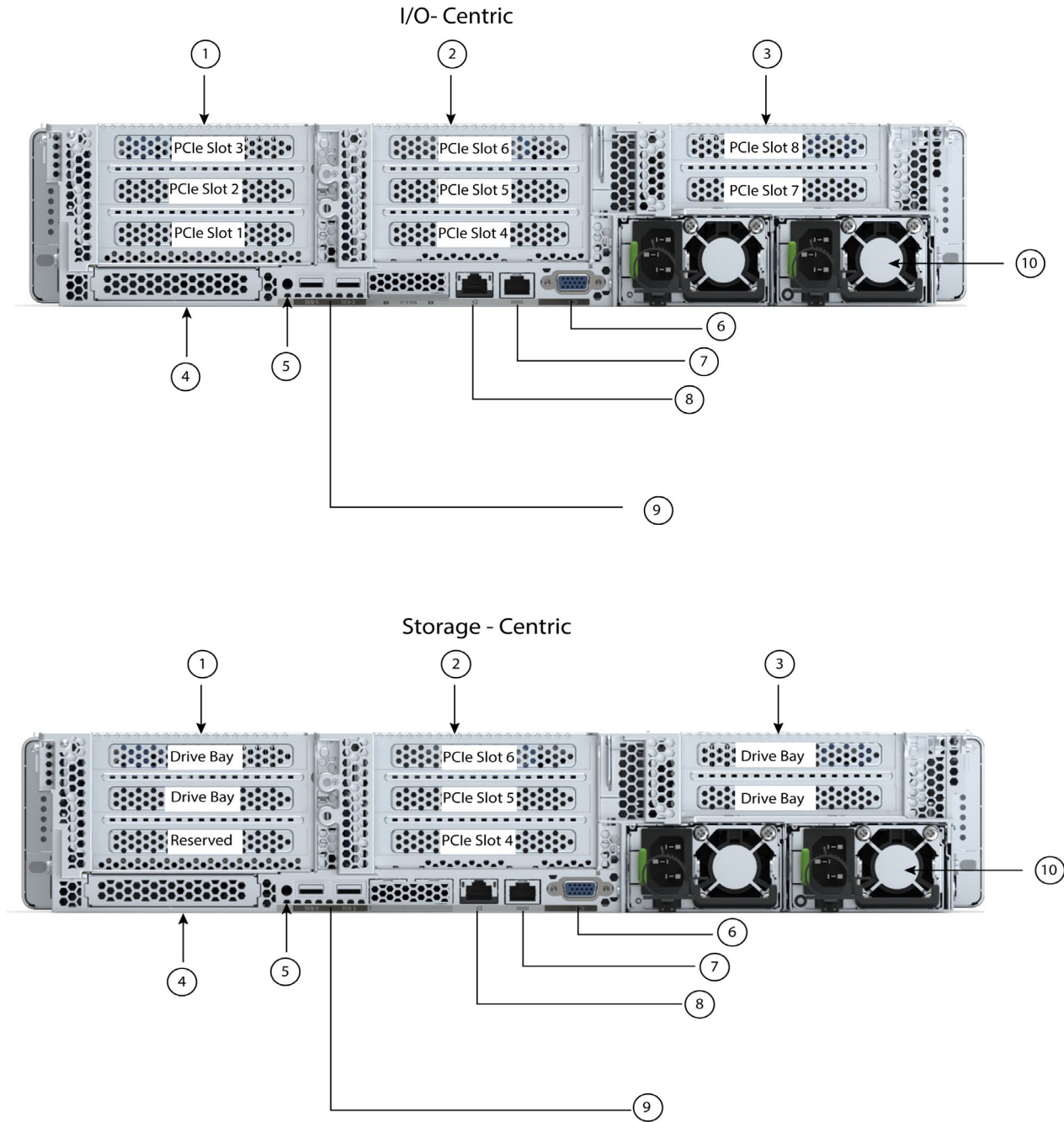
図 3 シャーシ背面図 (HXAF-E-245-M6SX)
