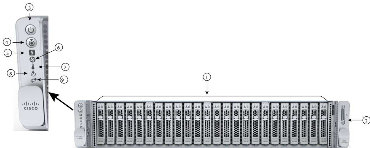
図 2 シャーシ前面図 (HXAF-E-245-M6SX)
