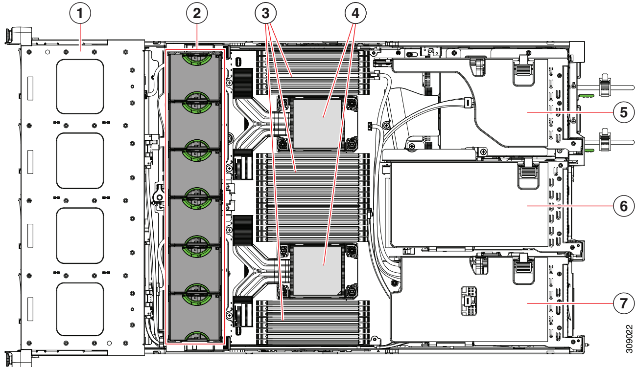
図 15 上部カバーを外した状態の Cisco HyperFlex HX245 M6 Edge All Flash およびハイブリッド サーバーノード
