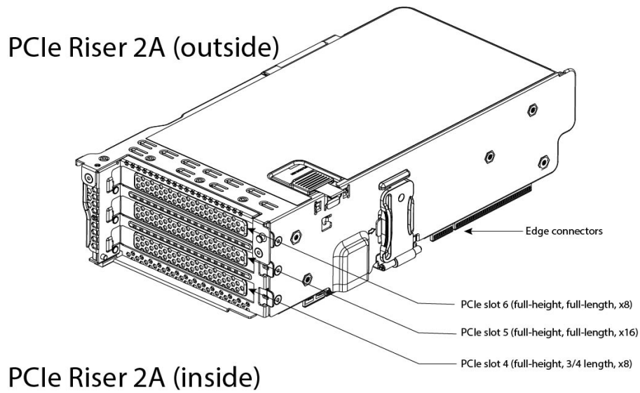
図 21 ライザー カード 2A
