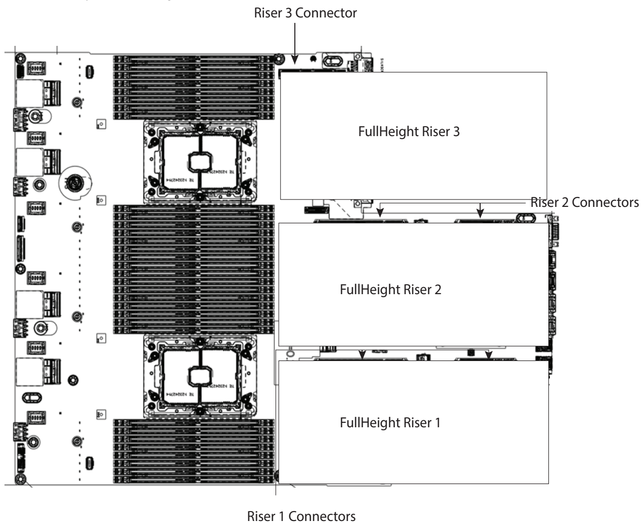
図 17 3 つのフルハイト ライザーが接続された HyperFlex HX245 M6 Edge All Flash/ ハイブリッド サーバー ノード
