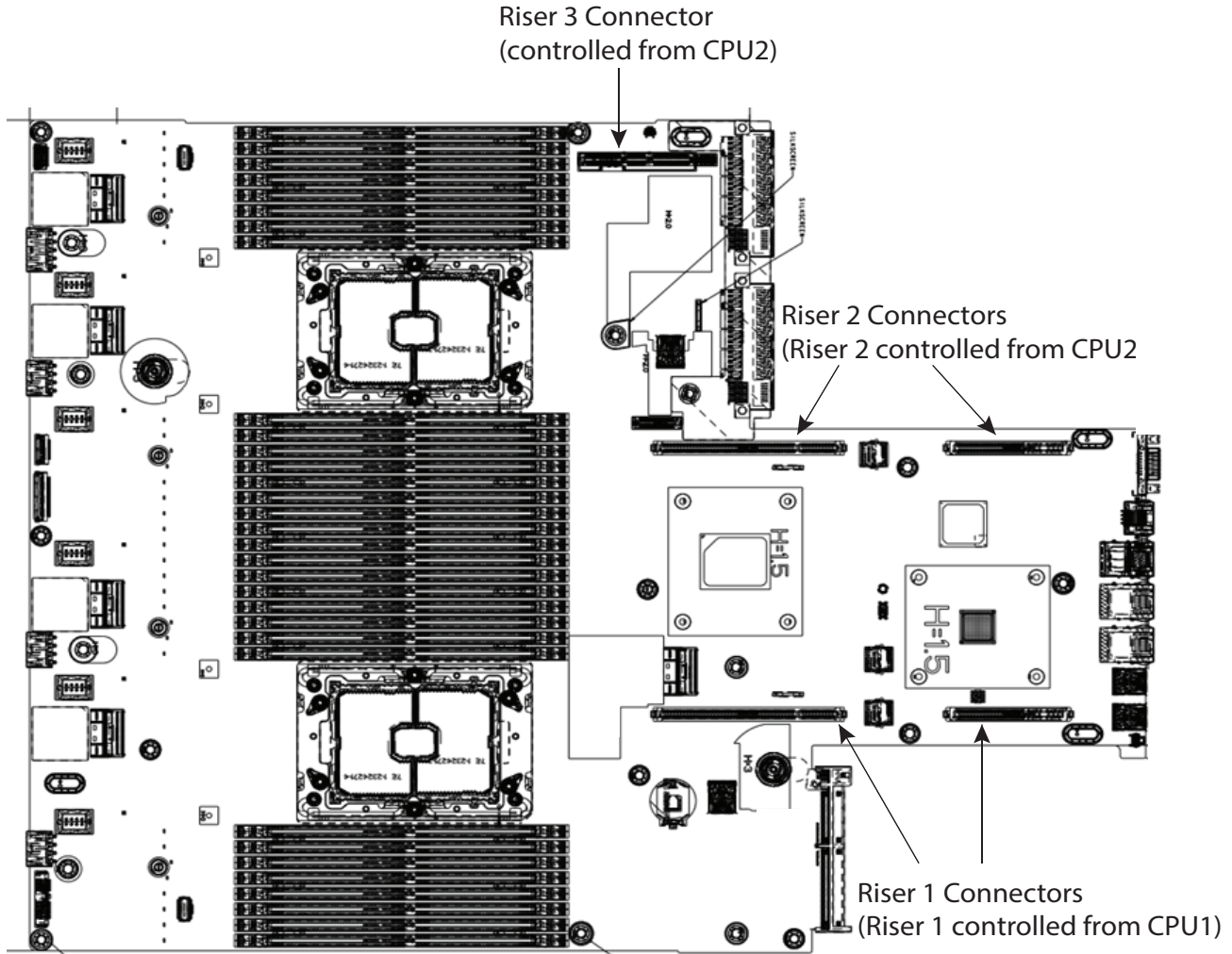
図 16 HyperFlex HX245 M6 Edge All Flash およびハイブリッド サーバー ノードのライザー コネクタの位置
