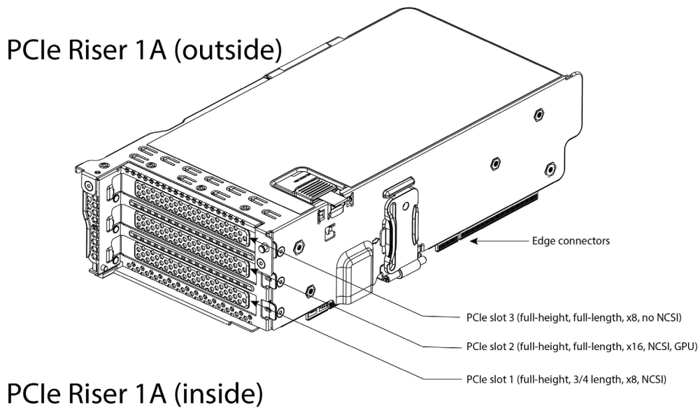
図 19 ライザー カード 1A
