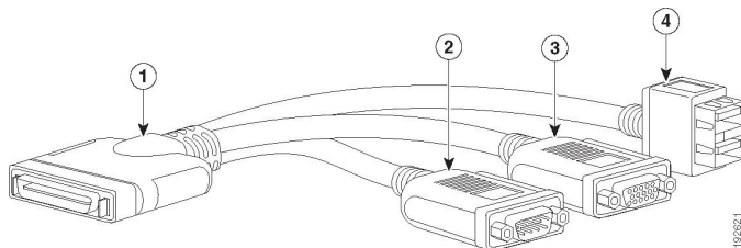
図 26 KVM ケーブル
