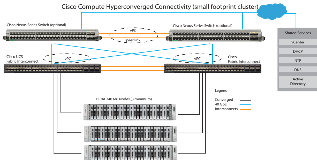
図 5 データセンター ファブリック インターコネクト展開モードの HCIAF240C M6 All-Flash サーバーを使用するスモール フットプリント クラスター
