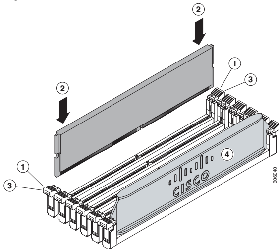
Figure 16 メモリの交換
