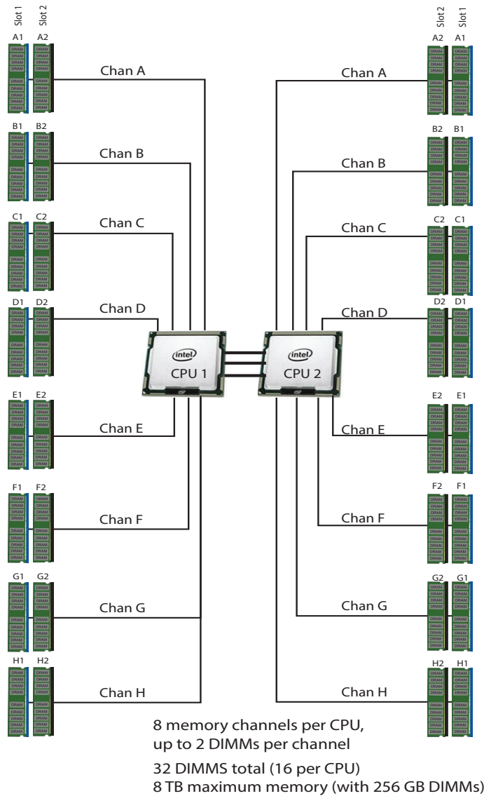
図 4 HCIAF240C M6 All-Flash サーバーのメモリ構成
