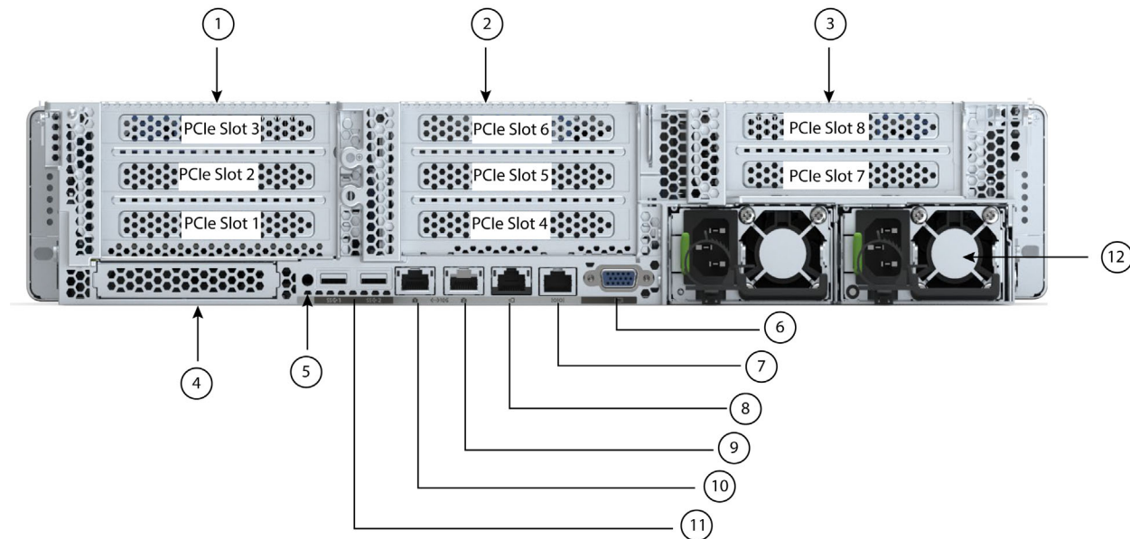
図 3 シャーシ背面図 : HCIAF240C-M6SX (All Flash)
