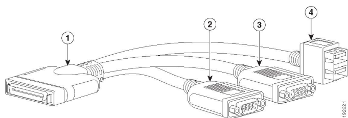
図 7 KVM ケーブル
