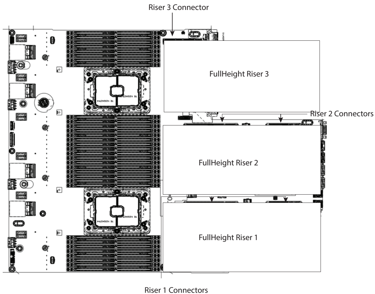
図 10 HClAF240C M6 All-Flash サーバー ライザー コネクタの位置
