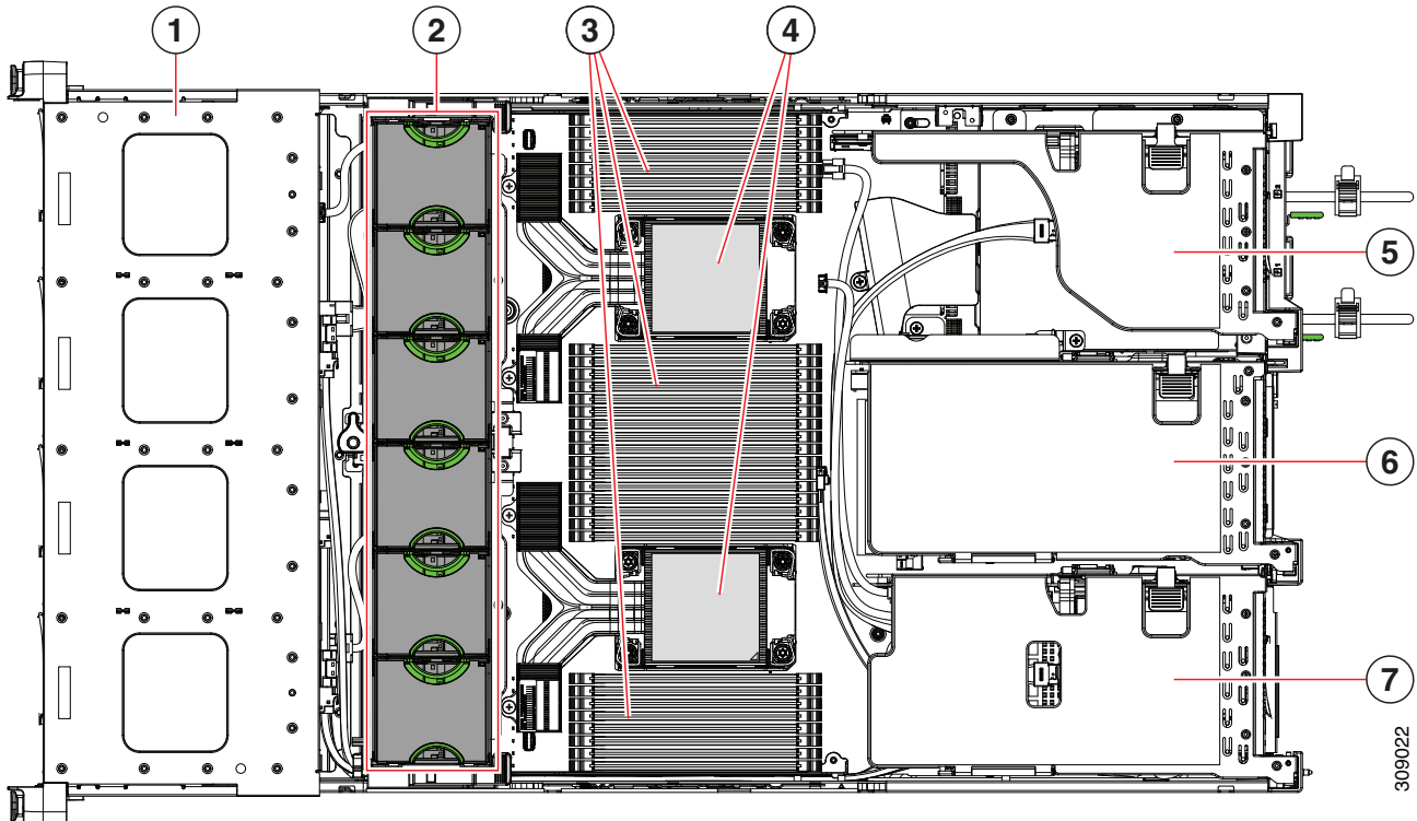
図 8 上部カバーを外した HCIAF240C M6 All-Flash サーバー
