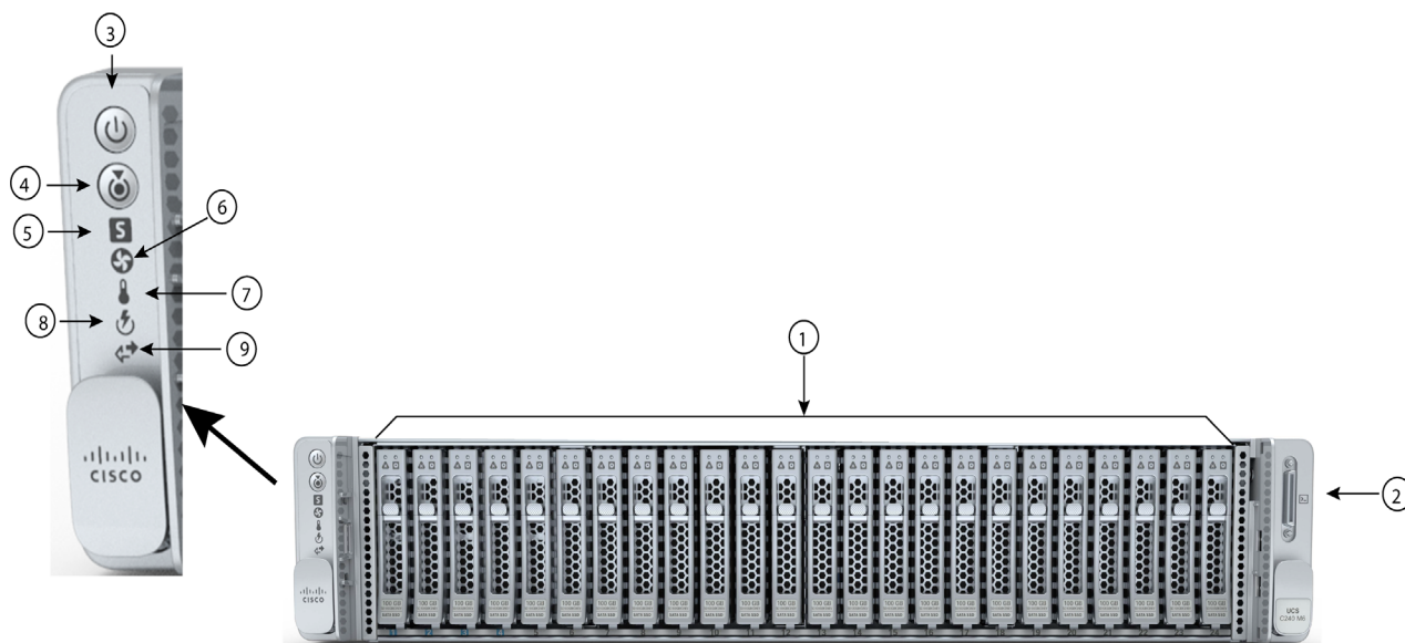
図 2 シャーシ前面図 - HClAF240C-M6SX (All-Flash)
